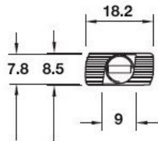
T-Bolt
