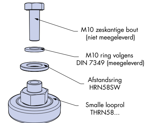
Doorganggat smalle looprol THRN58C/ENS met afstandring HRN58SW
