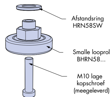
Blindgat smalle looprol HRN58C/ENS met afstandring HRN58SW
