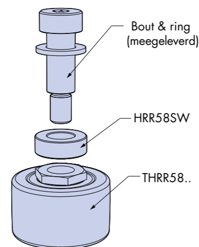
Doorganggat smalle looprol THRN58C/ENS met afstandring HRN58SW
